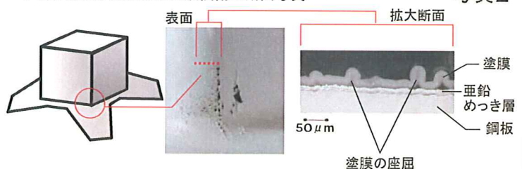
PCM 深絞り成形時の塗膜損傷の断面写真
