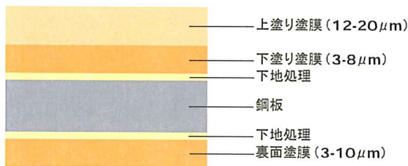
代表的なプレコート鋼板の構成 図6
