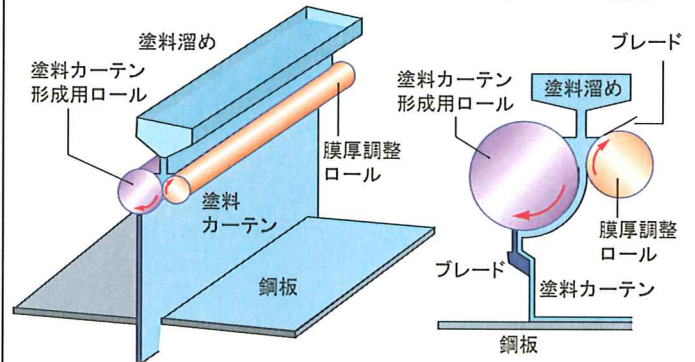
ローラーカーテンフローコーター 図8
