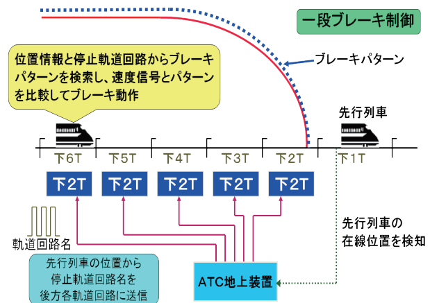
図2 デジタルATCによる制御
