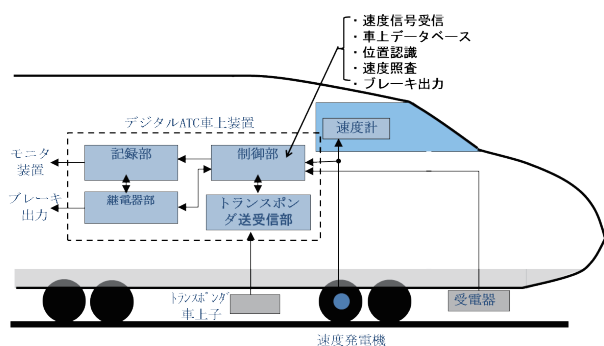
図3 デジタルATC車上装置構成
