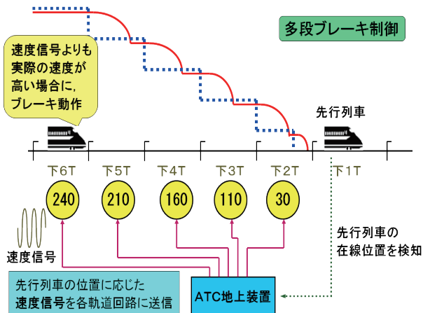
図1 アナログATCによる制御
